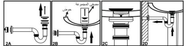
شكل 2. تركيب السيفون بدلو و شكل U
