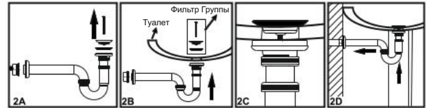
Рис 2. Монтаж сифона с чашкой и U-образной формы
