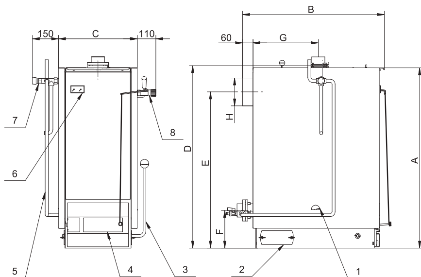
Obr. 1 Hlavní rozměry kotle SL14E, SL20E, SL27E
