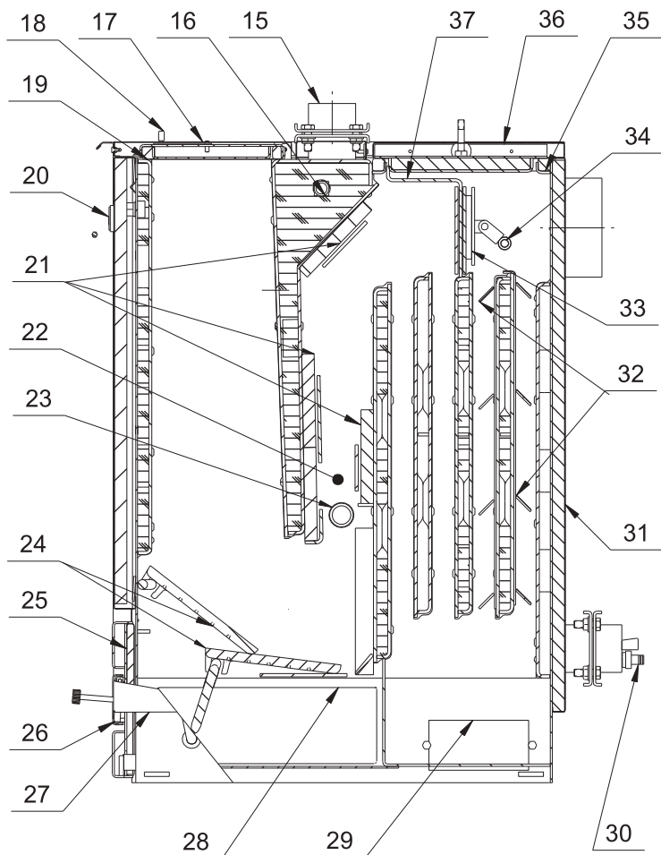
Obr. 4 Schéma kotle SL27E
