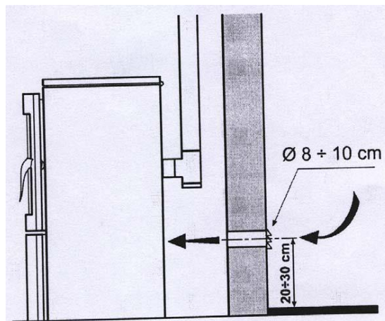
Obrázek 8. Minimální vzdálenost pro instalaci ventilační mřížky
