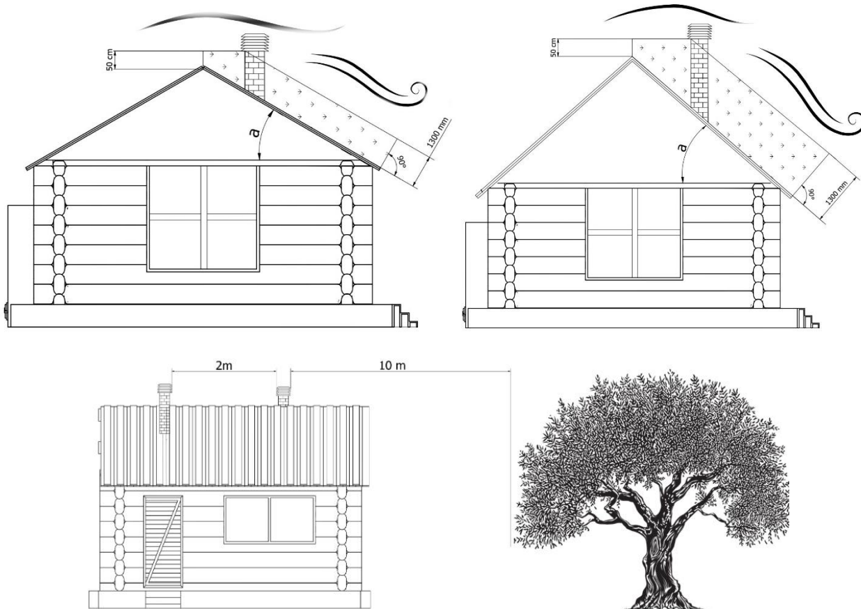
Komín - umístění a vzdálenost
