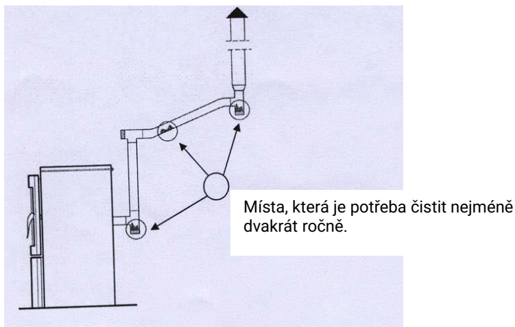
Obrázek 18. Místa, která je potřeba čistit nejméně dvakrát ročně
