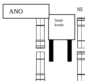
Obrázek 7. Způsob montáže kouřovodu
