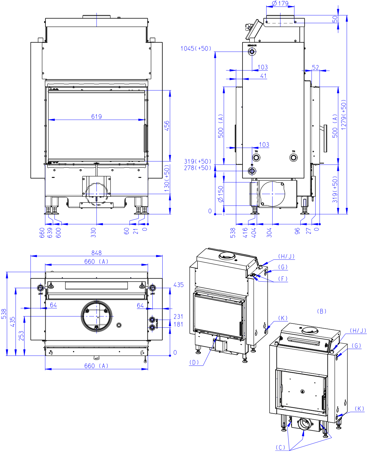
DWB2M 01P - Rozměrový náčrt, Rozmerový náčrt, Schemat wymiarowy, Размерный эскиз
