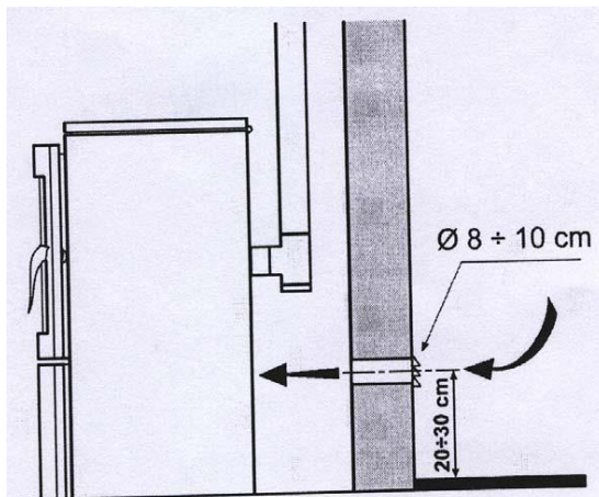
Obrázek 8. Minimální vzdálenosti pro instalaci větrací mřížky
