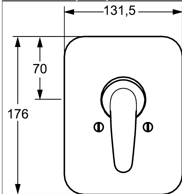
Výkres výrobku
