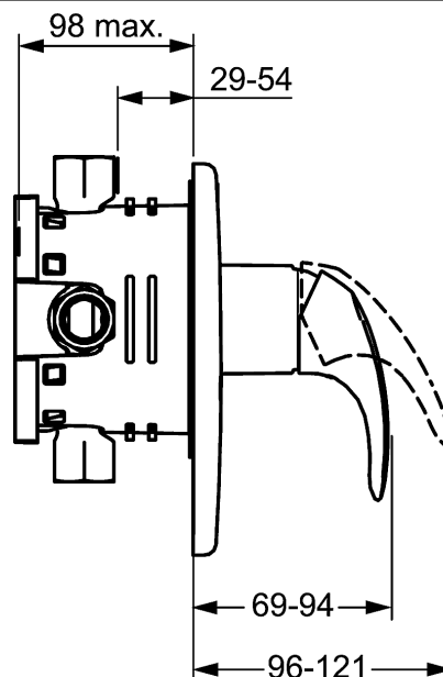
Výkres výrobku
