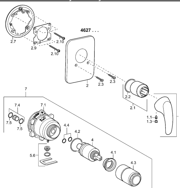
Výkres výrobku
