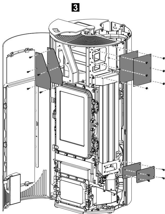
Obrázek 4: Demontáž boční stěny
